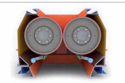
Řez drtičem DVU pro jemné drcení
