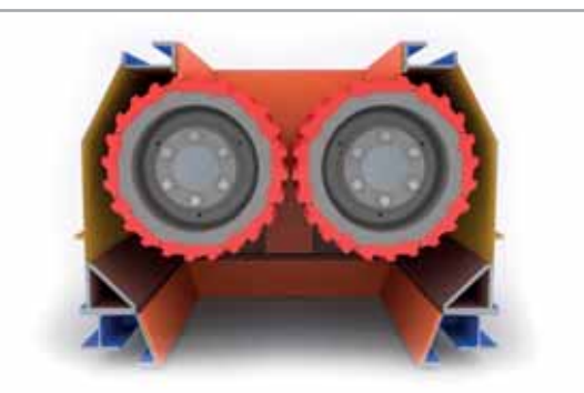
Řez drtičem DVU pro hrubé drcení
